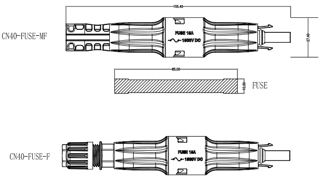
保险丝规格 CN40-FURY- ** FUSE Specification (2~30A)
