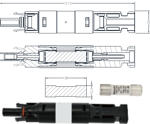
保险丝规格 CN40-FURY- ** FUSE Specification (2~30A)
